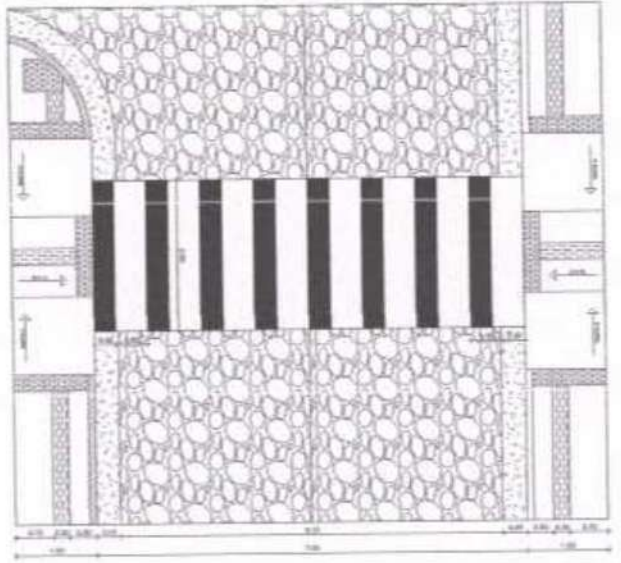
03) DETALHE TRANSVERSA
