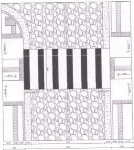
03) DETALHE PARA ELAVADA ESCALA: 1:20
