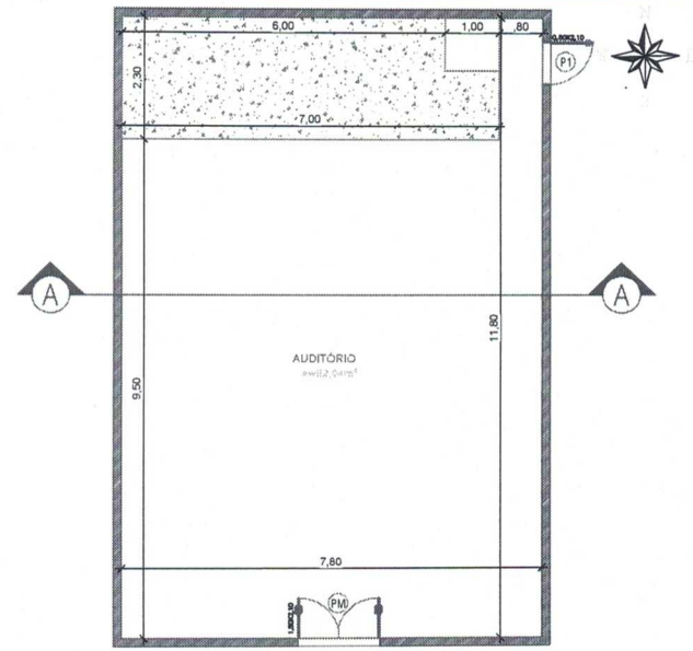
01 PLANTA BAIXA esc: 1:100
