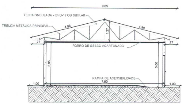
02 CORTE - AA esc: 1:100
